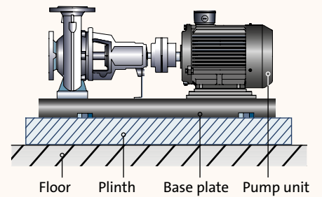
Fig. 2.1.7: Plinth
