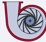
Fig. 1.1.18: Single-volute casing
